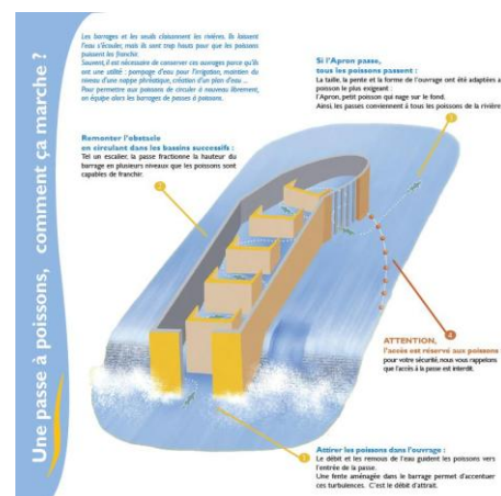
Figure 4 : Schéma d'une passe à poisson
