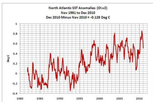
Figure 7 : Graphique représentant la variation de température du nord de l'Atlantique au cours du temps
