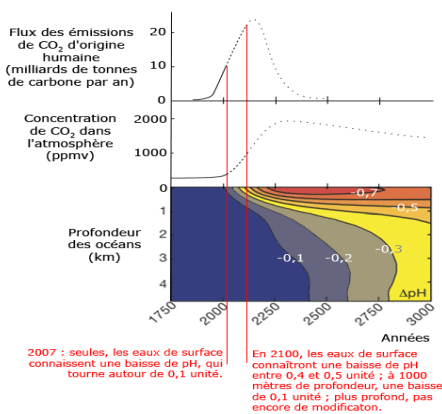
Figure 2 : Graphique représentant l'acidité des océans en fonction de la profondeur et du taux de CO 2 atmosphérique émis par l'homme
