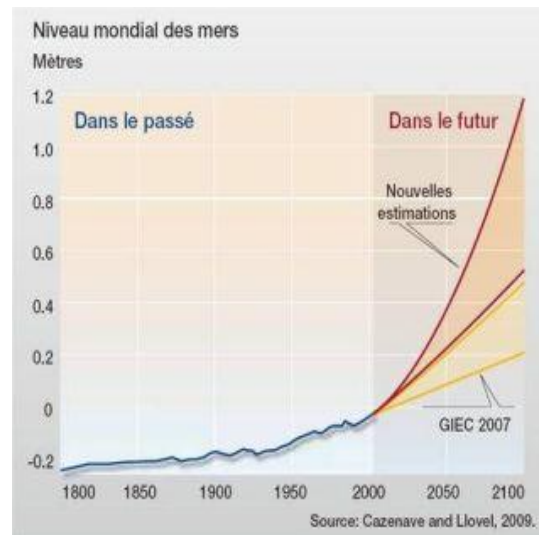
Figure 3 : Graphique représentant le niveau des mers dans les années passées et modélisant les niveaux des mers pour le siècle à venir
