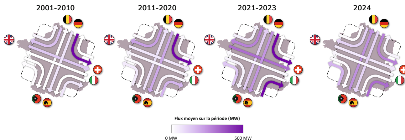
Figure 1 – Évolution des flux traversant le système électrique français au cours des dernières décennies (moyennes au cours de la période considérée)
