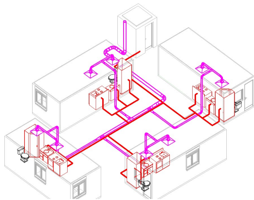
Tracé des réseaux sur la maquette 3D
